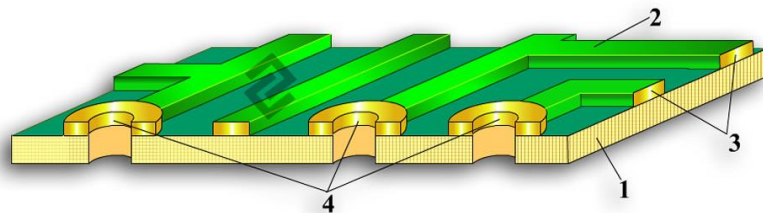
Рисунок 4 – Конструкция односторонней печатной платы: 1. Диэлектрик; 2. Защитный слой (маска); 3. Токопроводящая дорожка; 4. Контактное отверстие;
