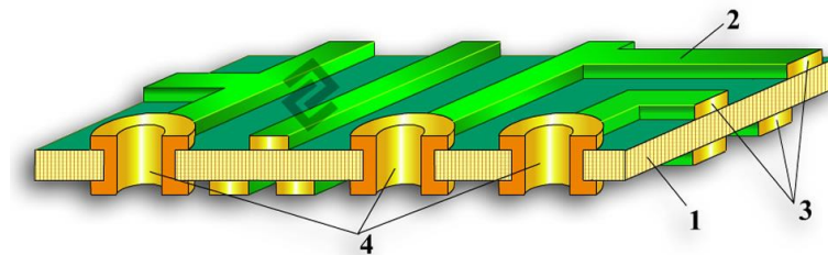
Рисунок 5 – Конструкция двухсторонней печатной платы: 1. Диэлектрик; 2. Защитный слой (маска); 3. Токопроводящая дорожка; 4. Контактное отверстие;
