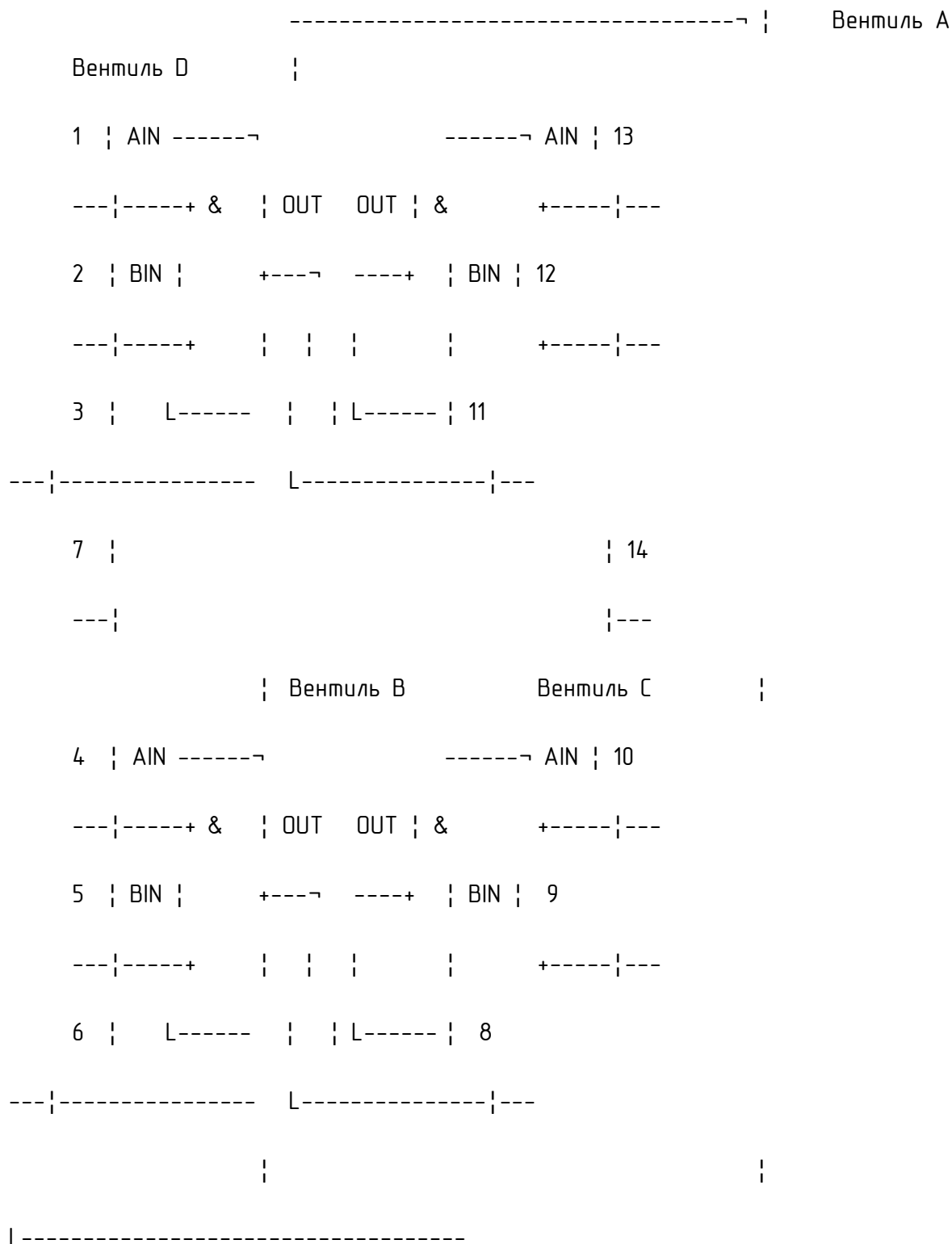
Рисунок 4 - Упаковка вентилей в корпусе
