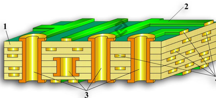
Рисунок 6 – Конструкция многослойной платы: 1. Диэлектрик; 2. Защитный слой (маска); 3. Контактное отверстие; 4. Токопроводящая дорожка;
