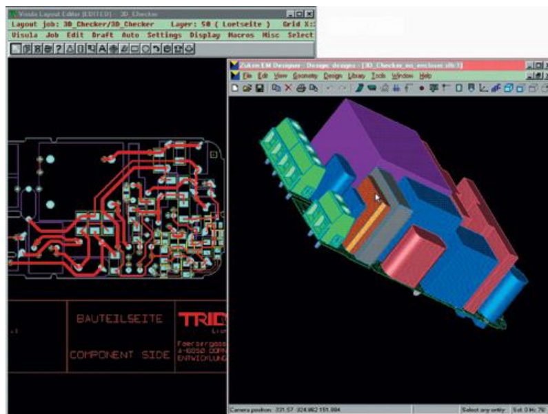
Рисунок 1.3 - Трёхмерное моделирование платы средствами компании Zuken
