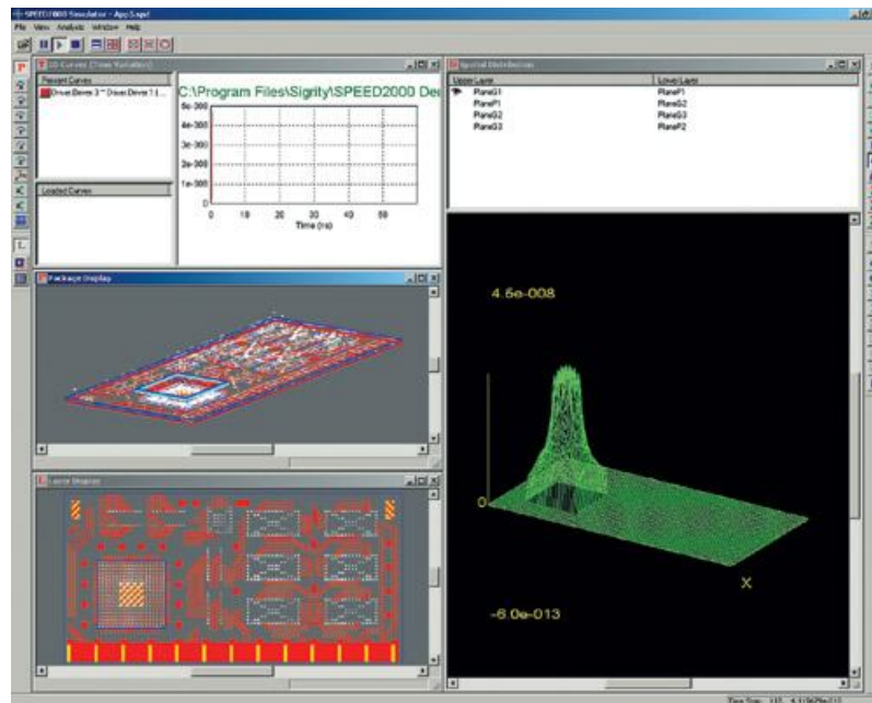
Рисунок 1.4 - Анализ помех в слое заземления в пакете Speed 2000 компании Sigrity
