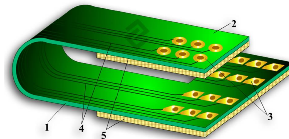
Рисунок 8 – Конструкция гибкожестких печатных плат: 1. Диэлектрик (Полиамид); 2. Защитный слой (маска); 3. Контактное отверстие; 4. Токопроводящая дорожка; 5. Жёсткая подкладка;
